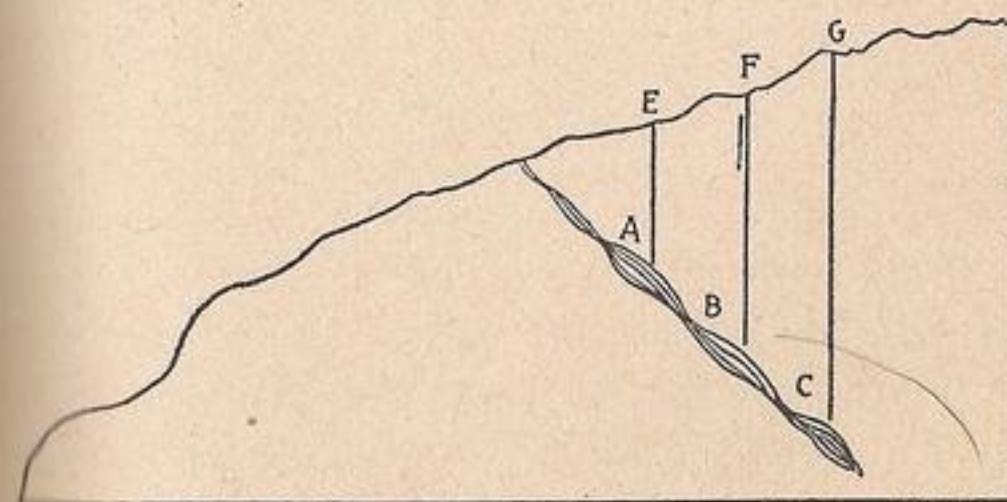
Pinchout Vein.
